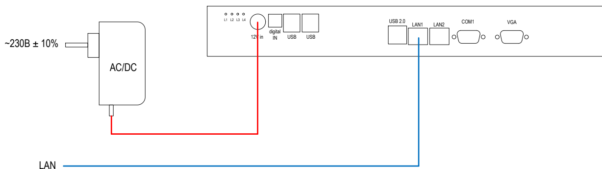
Терминал типа SPC-15GI.
