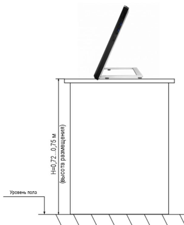
Терминал типа SPC-15GI
